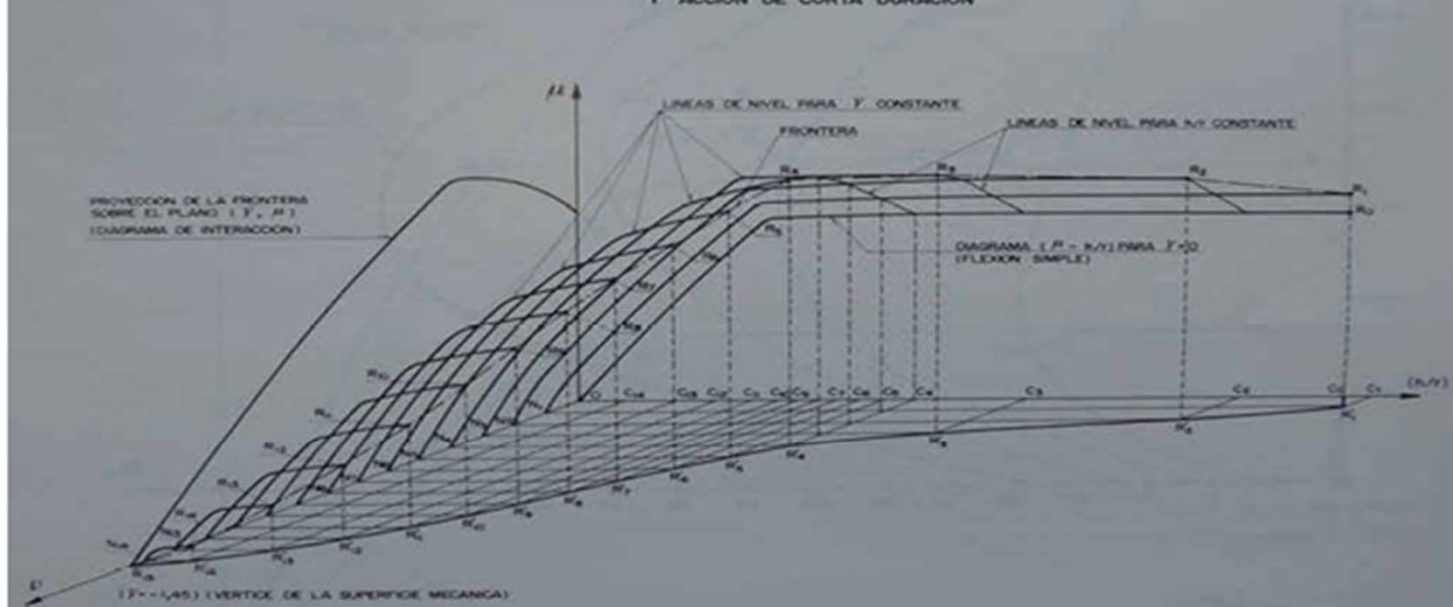
Fig. 2. Superficie mecánica de una sección de hormigón armado según Juan José Arenas: De su libro sobre soportes (1980)
